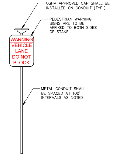
HAUL ROAD 100' LANE MARKER SCALE: N.T.S
